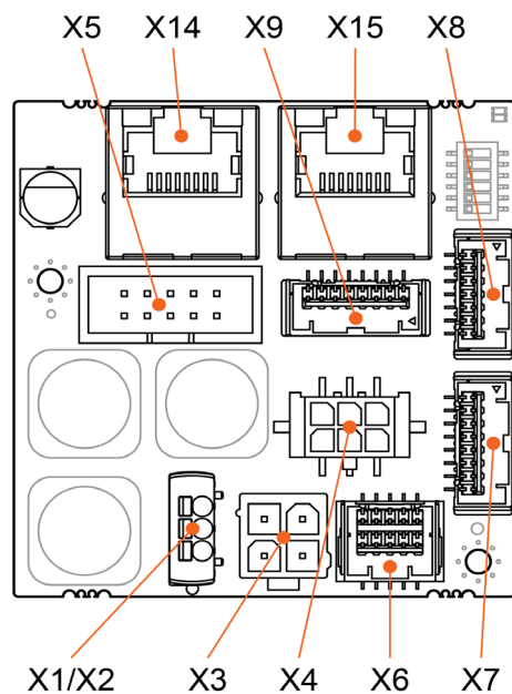
図 3-14 EPOS4 CB 50/5 – 接続
